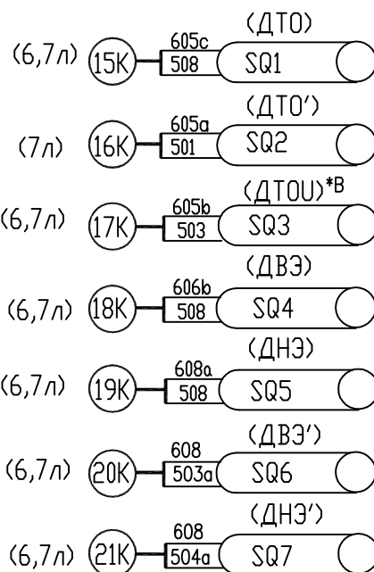
Вариант подключения ГВУ УКЗ-ВТ
